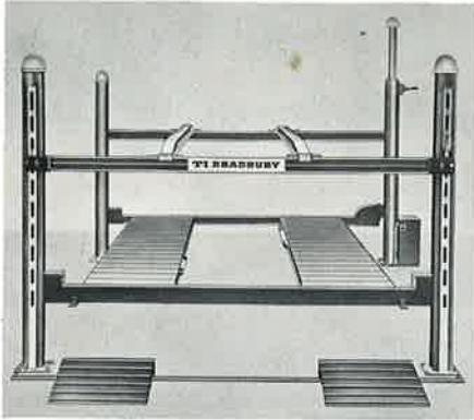
773A 'Dockmaster' 4 post lift 3½ tonnes.
